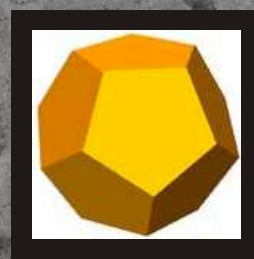
Sólidos Platónicos
